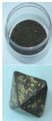
砂鉄 磁鉄鉱の結晶
