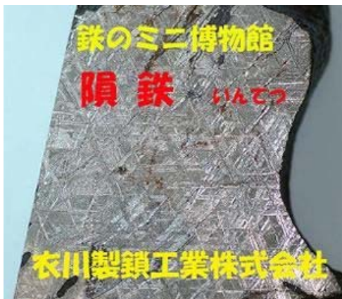
隕鉄 ナミビア共和国産
